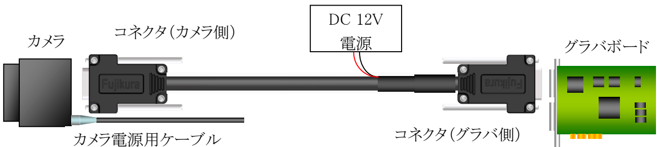
図 1 接続図 (Base Configuration)
