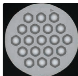
マルチコアファイバ(19コア)
