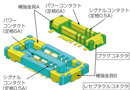
図1 コネクタ外観図
