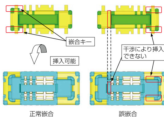
図2 嵌合キー構造
