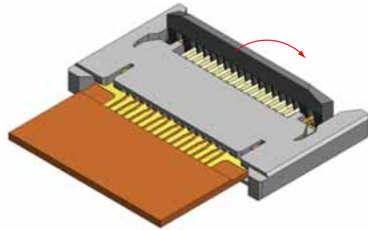
図2 回転バックロック機構
