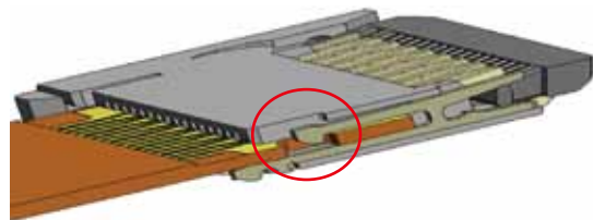
図3 ケーブルロック機構
