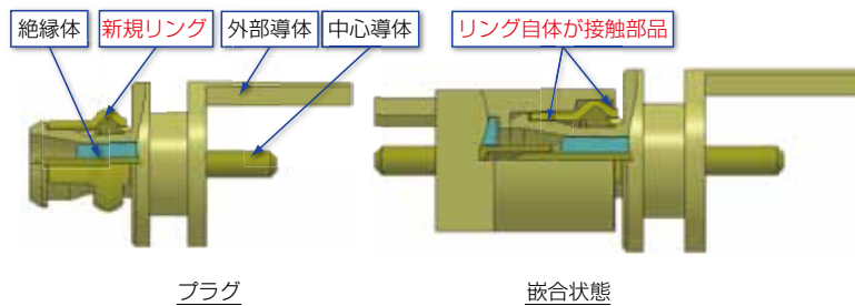
図2 MMCXFシリーズ
