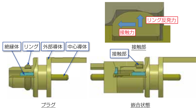
図1 MMCXシリーズ (従来品)
