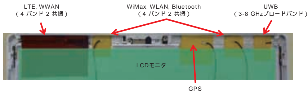
図1 ノート PC 実装例 (薄緑は LCD 部)
