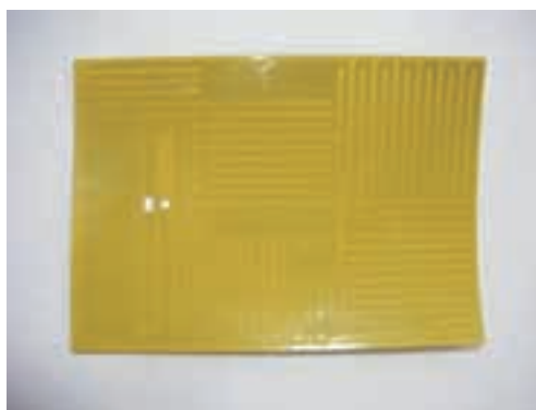
図2 TV 受信用アンテナ
