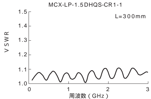
図 1 VSWR
