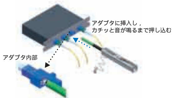
図3 アダプタ内のフェルル端面清掃
