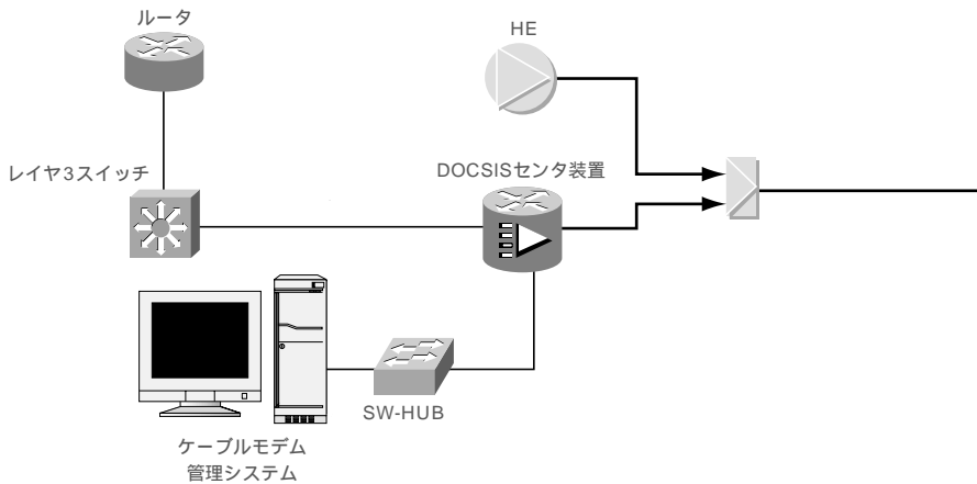
図1 システム構成例
